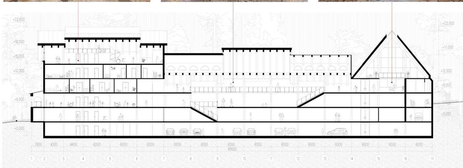
Продольный разрез
