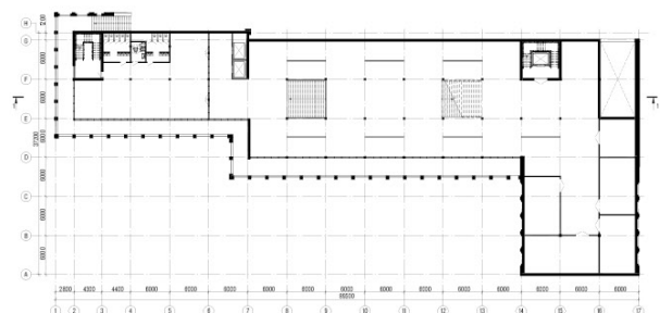
ПЛАН 1-ГО ЭТАЖА
