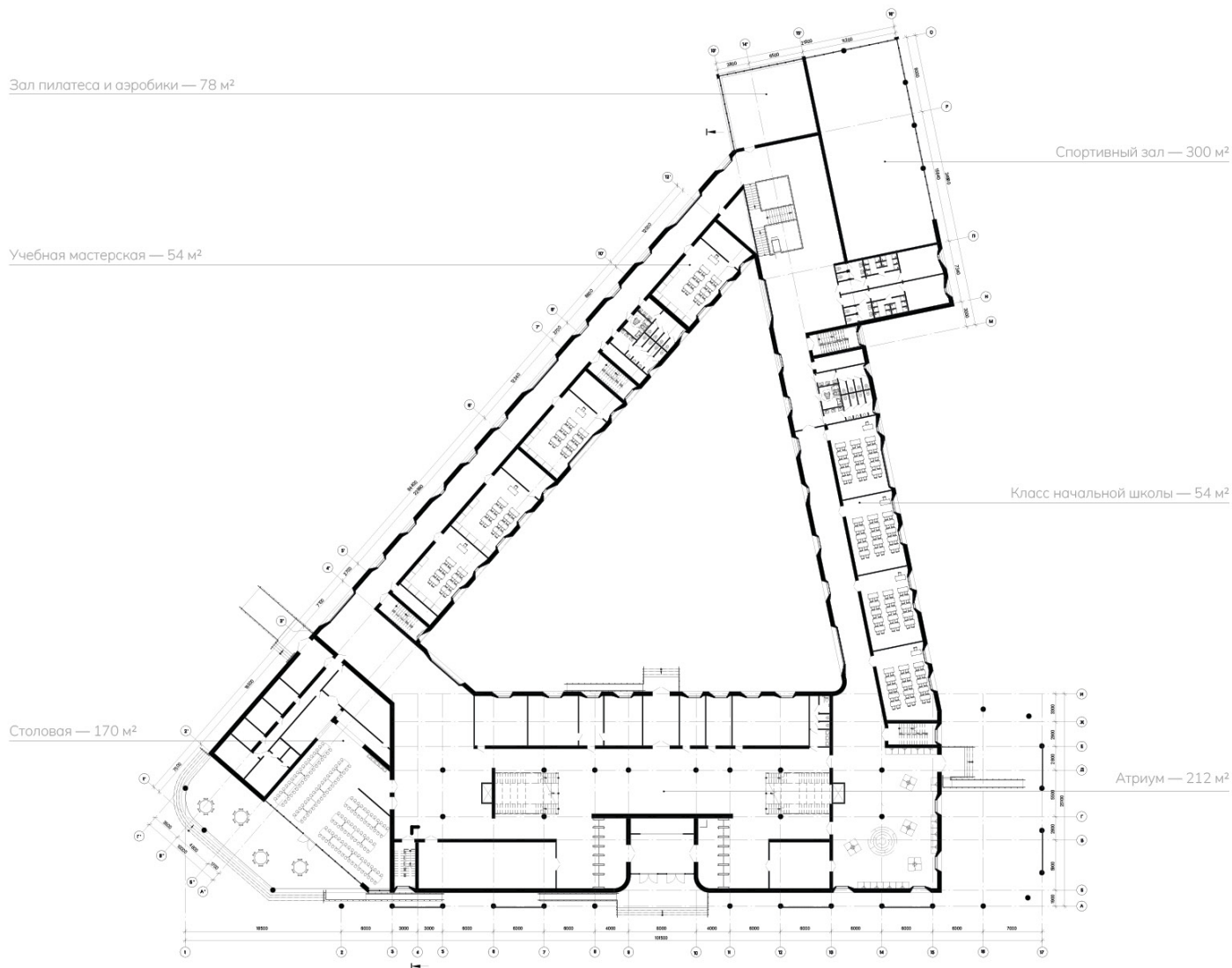
План первого этажа
