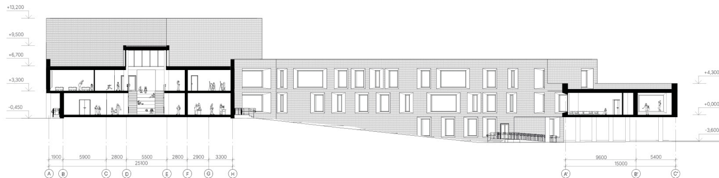
Разрез здания
